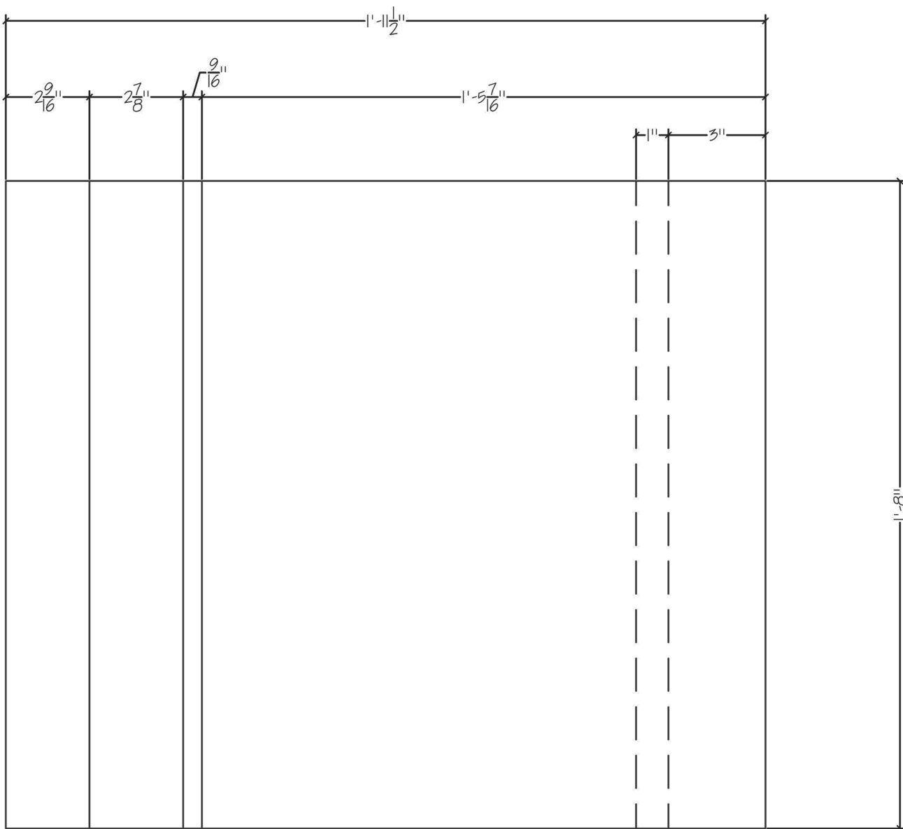
① PLAN SCALE: 3" = 1'-0"
